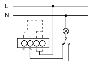
1 Gang, 2 Way
