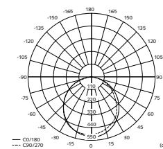
99 700 11: Ljufördelningskurva
