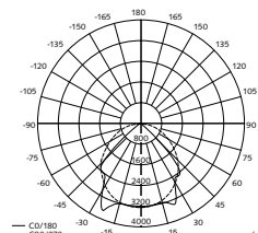
72 972 52: Ljufördelningskurva
