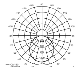
70 137 03: Ljustfördelningskurva
