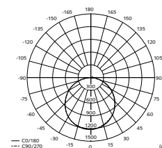
99 700 09: Ljusfördelningskurva
