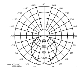
70 137 04: Ljustfördelningskurva
