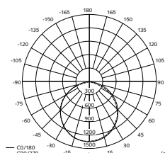
70 137 02: Ljustfördelningskurva
