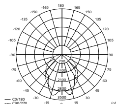
72 972 51: Ljufördelningskurva
