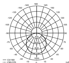
99 700 04: Ljusfördelningskurva
