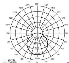
99 700 08: Ljusfördelningskurva
