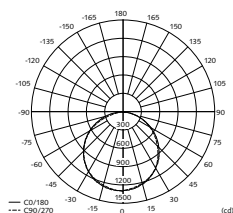
99 700 05: Ljusfördelningskurva
