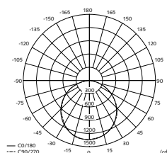
70 137 01: Ljustfördelningskurva
